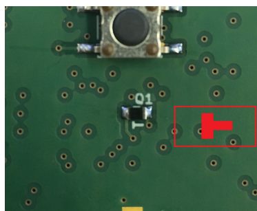
Abbildung 3: Polarität des Fototransistors
