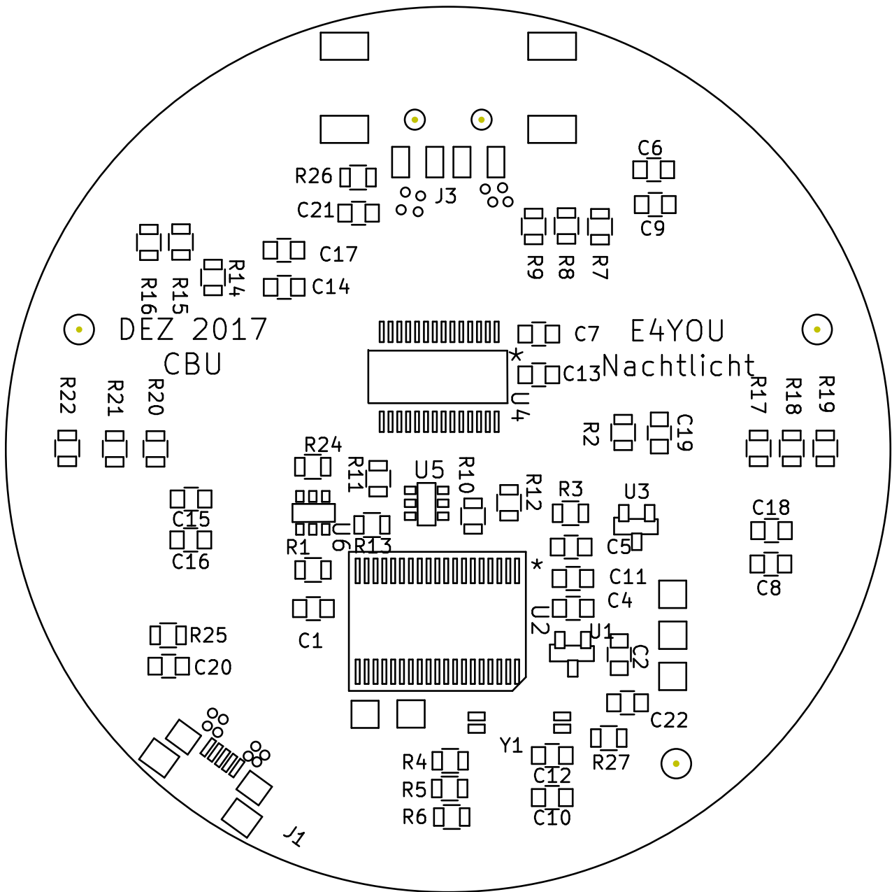
Abbildung 4: Bestückungsplan Unterseite
