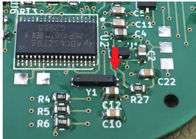
Abbildung 5: Ausrichtung des Quarz
